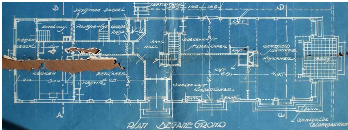
Afb. 16 De enigszins beschadigde tekening van de begane grond.
