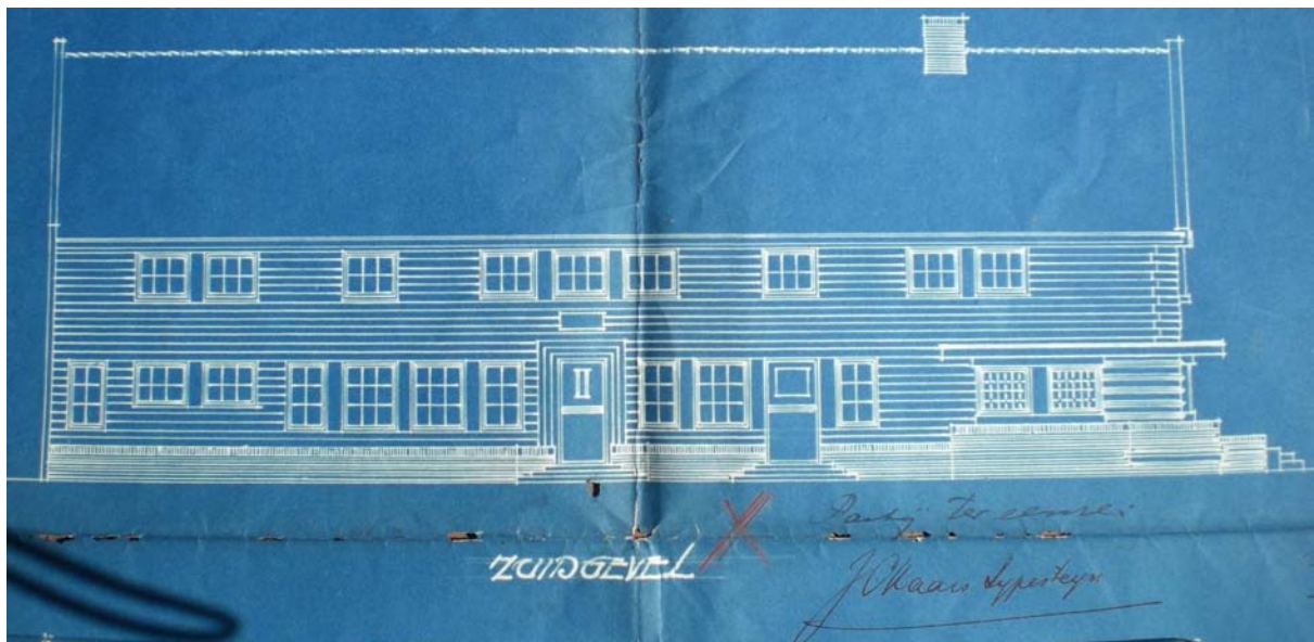
Afb. 12 Het ontwerp van de zuidgevel van het Weversend. Het houten gevelbord heeft in de bestektekening al een plaats gekregen. Op de tekening, die onderdeel vormde van het bestek is de handtekening van Jan Kaars Sijpesteijn te lezen.
