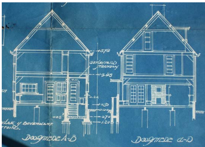
Afb. 17 Doorsnede A-B tpv de keuken en C-D tpv de woonkamer, met de funderingsprincipes. Ter ondersteuning van de vloerbalklaag zijn bij doorsnede C-D twee brede funderingen getekend, die duiden op putringen. De paalfundering onder de bloembakken en de stookkelder zijn duidelijk afwijkend getekend.
