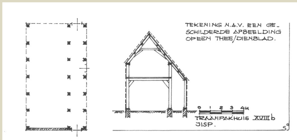
Tekening van een traanpakhuis in Jisp Tekening door S. de Jong
